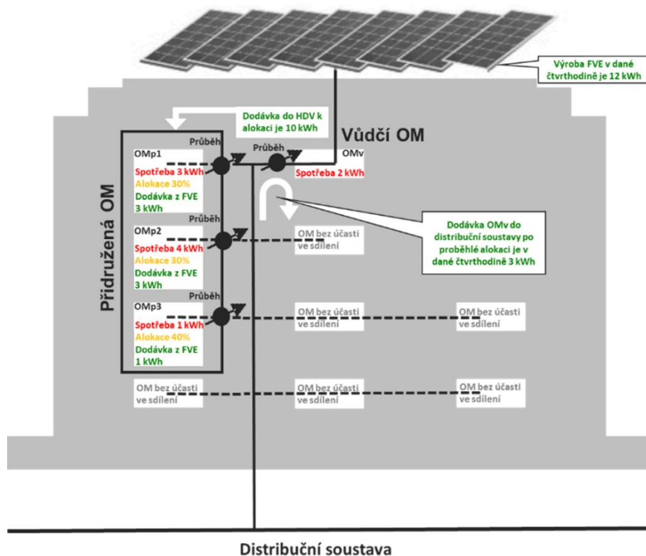
Obrázek 26: Schéma výroby elektřiny v bytovém domě a její rozdělení mezi jednotky
